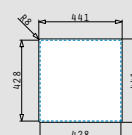
Flächenbündiger Einbau
