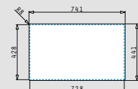
Ausfrässhablone beiliegend
