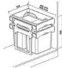
3-fach Trennung Abmessungen: 339 x 486/985 x 428 mm
