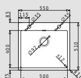
Beihaltete Ablaufgarnitur
