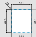
Flächenbündiger Einbau
