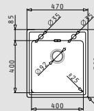
Beinhaltete Ablaufgarnitur
