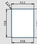
Flächenbündiger Einbau
