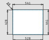
Flächenbündiger Einbau
