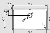
Beihaltete Ablaufgarnitur
