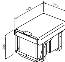
3-fach Trennung Abmessungen: 355 x 470 x 365 mm
