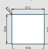
Flächenbündiger Einbau
