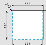
Flächenbündiger Einbau
